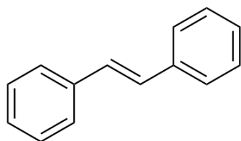
stilbene
